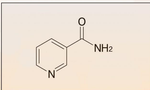
Niacinamide ( C_7H_6O_3 )
